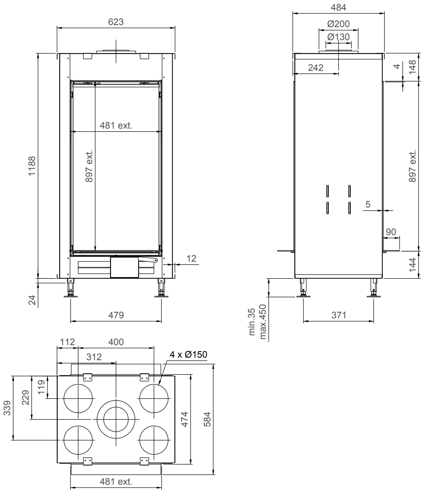
True Vision 550DV - Type 2 - 90mm
