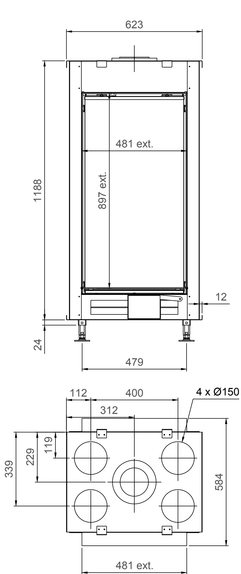
True Vision 550DV - Type 3 - 60mm
