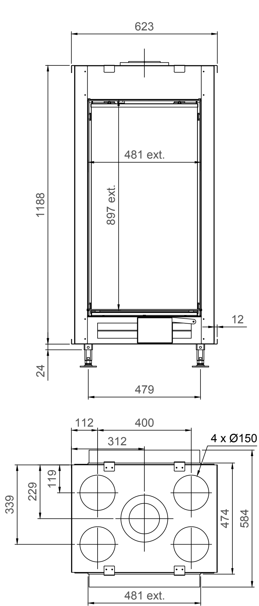
True Vision 550DV - Type 2 - 60mm
