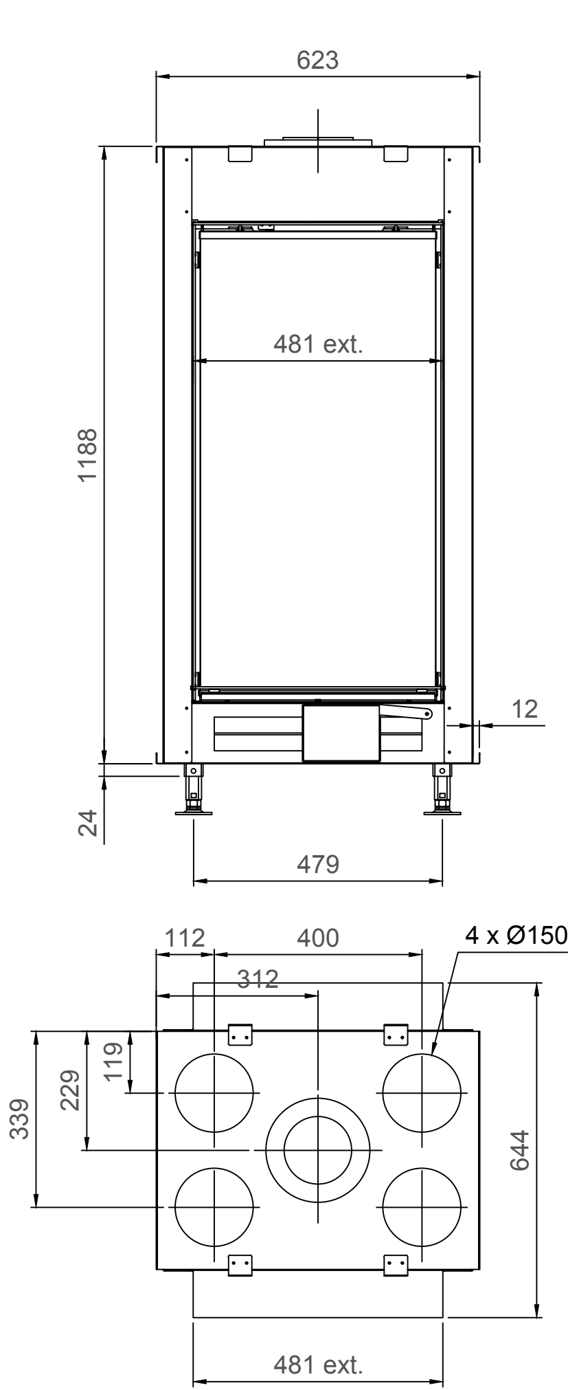
True Vision 550DV - Type 3 - 90mm
