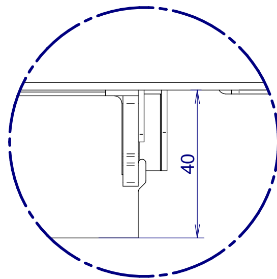
DETAIL A 1:1
